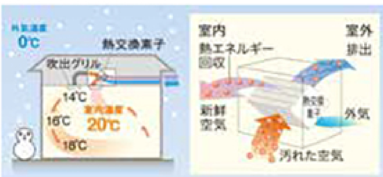
■熱交換換気のしくみ(冬期の場合)
